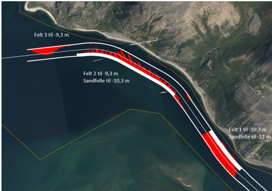
Govva 38: Oppalašeanadat čiekŋudanguovllus válljejuvvon molssaeavttus (kombinašuvdnamolssaeaktu).
