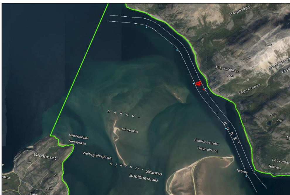
Govva 28: Oppalašeanadat mearraguovlluin, maidda molssaeavttu OB čuovvu bajásdoalločiekŋudeapmi jáhku mielde váikkuhivččii. Sáhcut merkejit plánejuvvon ođđa fávlelinnjema, eai dáláš. Gáldu: Multiconsult.
