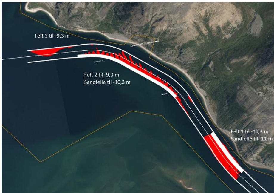
Govva 30: Oppalašeanadat čiekŋudanguovllus válljejuvvon molssaeavttus. Čiekŋudanguovllu lea merkejuvvon ruoksádiin ja sáttojorpmiit vielgadiin, Vilges sáhcut čujuhit 120 mehtera govdat fávlli ravdasárgáid ja gaskalinjá. Kárta ii leat mihttolávas.
